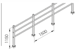
M12 GALVANISERET STÅL
